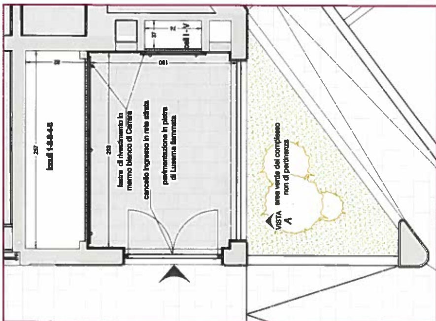
pianta TF1
