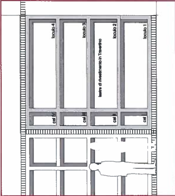
prospetto
