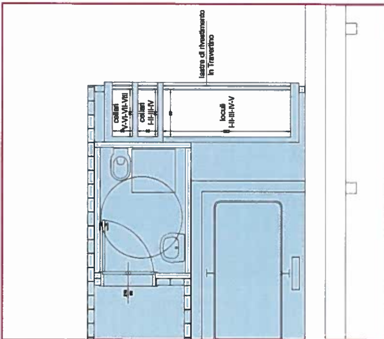
pianta TF10
