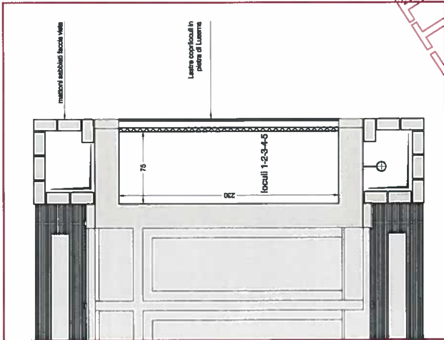
prospetto
